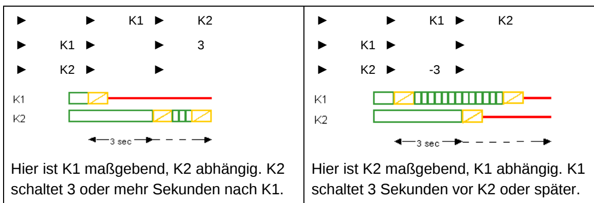
Abb. 4: Fester Ende-Versatz
