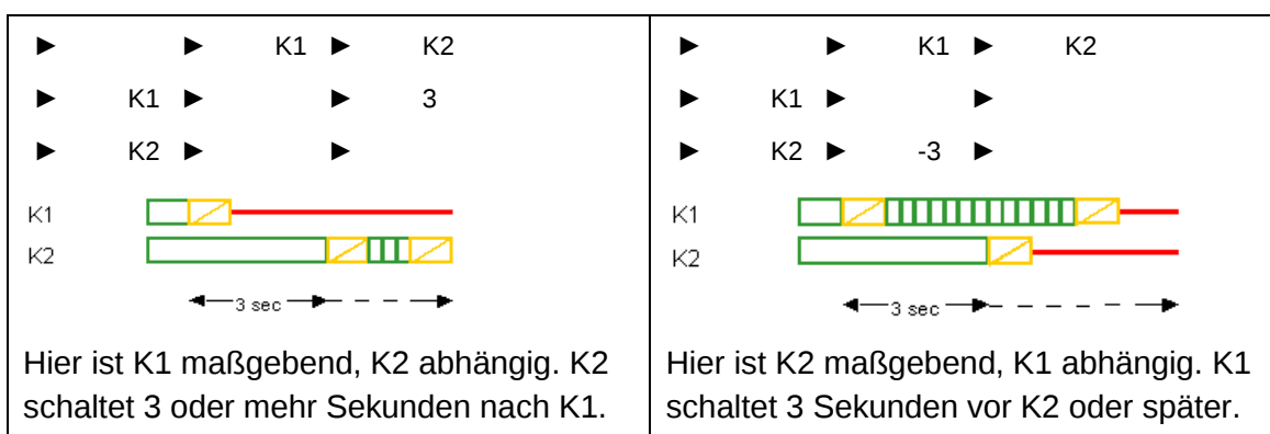
Abb. 5: Variabler Ende-Versatz
