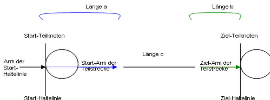
Abb. 10: Teilstreckenlänge
